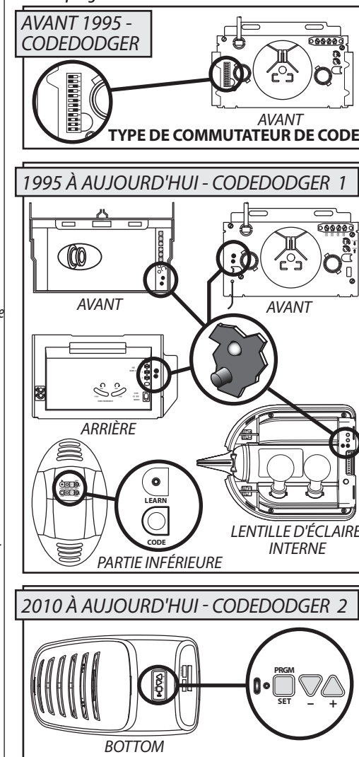
FIG. 1 TETE MOTORISÉE (pour divers modèles) Le cercle indique l'emplacement du commutateur de code de programmation et de la diode.
