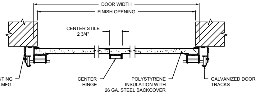
SECTION A-A
