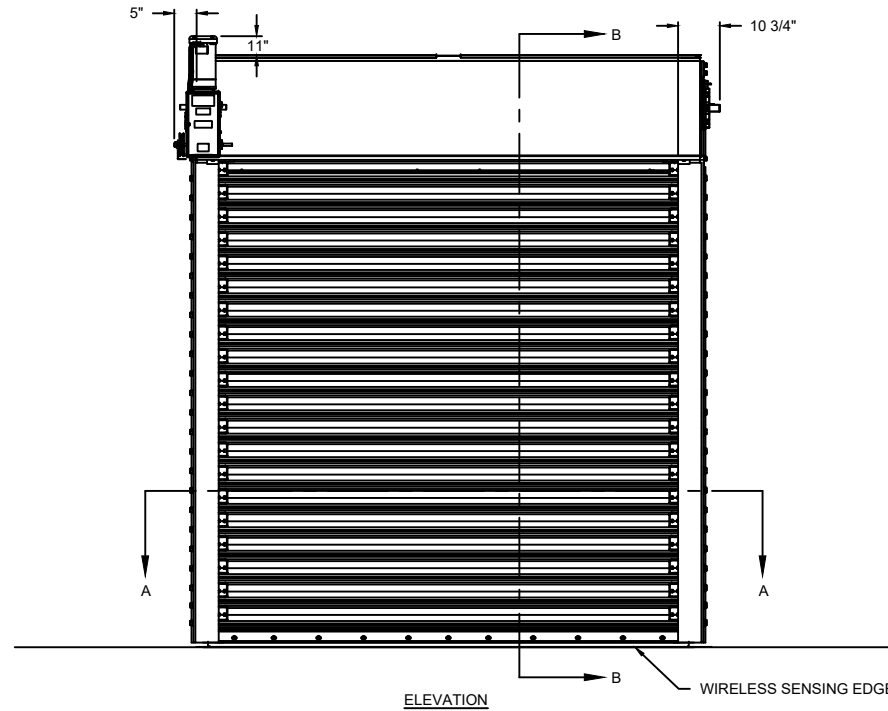
ELEVATION
